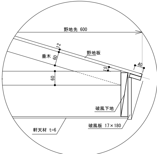
※2 軒先 納まり
