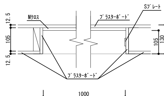
※ニッチ内部は全面クロス仕上げ
