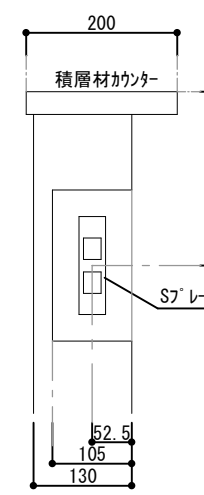
キッチン ニッチ 断面図
