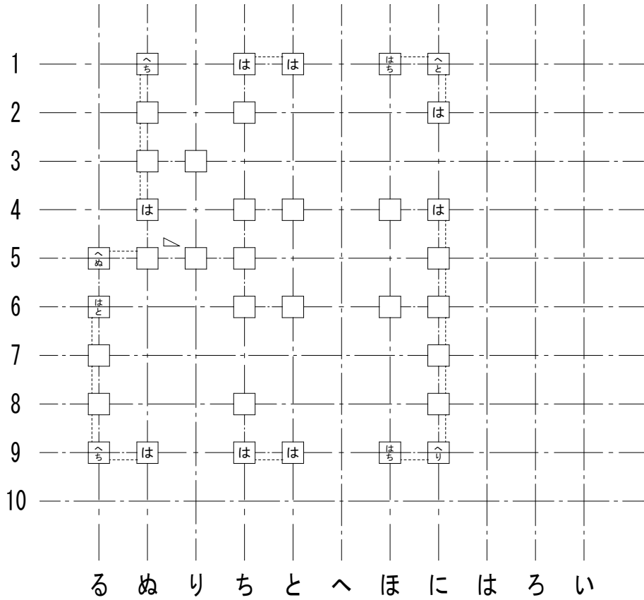
2階柱壁伏図
