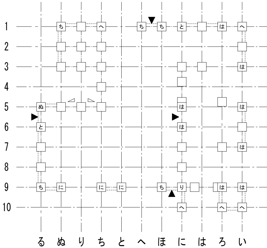
1階柱壁伏図
