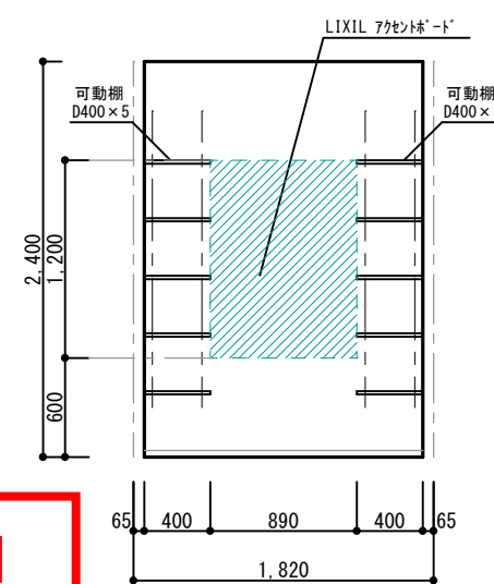
ハントリー 東面
