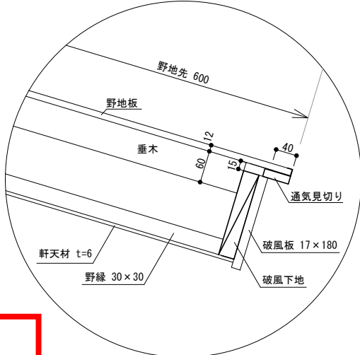
※3 軒先 納まり
