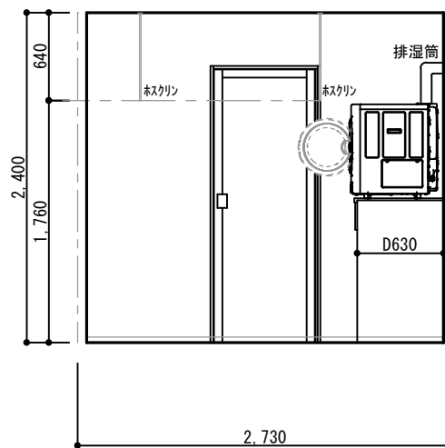
脱衣ランドリー 北面
