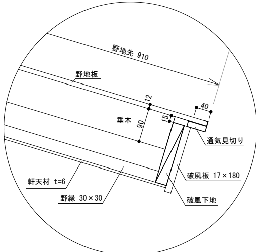
※1 軒先 納まり
